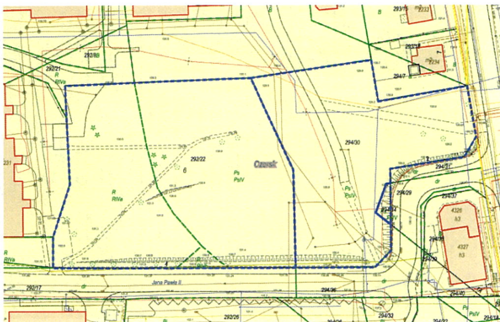
Rys. 4. Usytuowanie systemów infrastrukturalnych i klasoużytki
